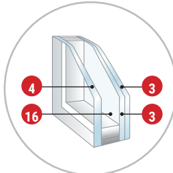
Vetrata SICURTHERM*
